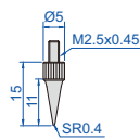
указательный наконечник
