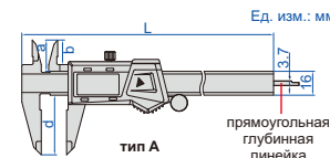
тип А прямоугольная глубинная линейка
