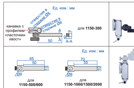
держатель тестового индикатора циферблатного типа (в комплекте)
