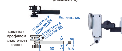
держатель тестового индикатора циферблатного типа (в комплекте)
