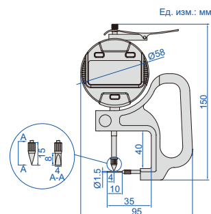
измерение толщины стенки или канавки
