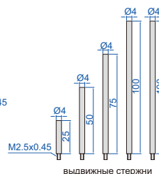
выдвижные стержни
