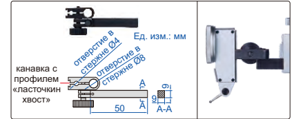
держатель тестового индикатора циферблатного типа (в комплекте)
