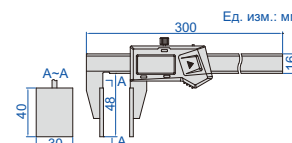
измерение диаметра резины, губки и т.д.
