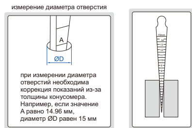
измерение диаметра отверстия
