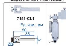
держатель тестового индикатора циферблатного типа (опция)
