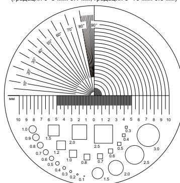
масштаб 7527-D2 (градация 0-5 мм: 0.1 мм, градация 5-10 мм: 0.5 мм)
