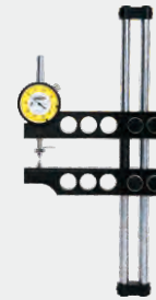
ПРИБОРЫ ДЛЯ ИЗМЕРЕНИЯ КОНУСНОСТИ РЕЗЬБЫ
