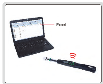
дальность передачи составляет 10 метров (без препятствий и электромагнитных помех)
